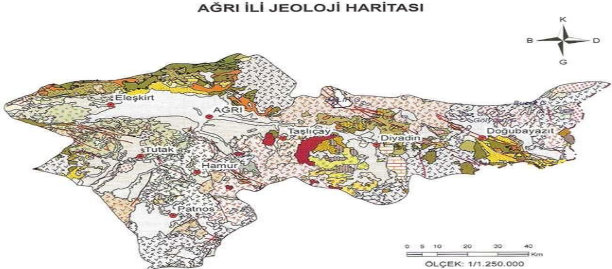
Şekil 1. Ağrı İli Genel Jeoloji Haritası (MTA, 2002).
